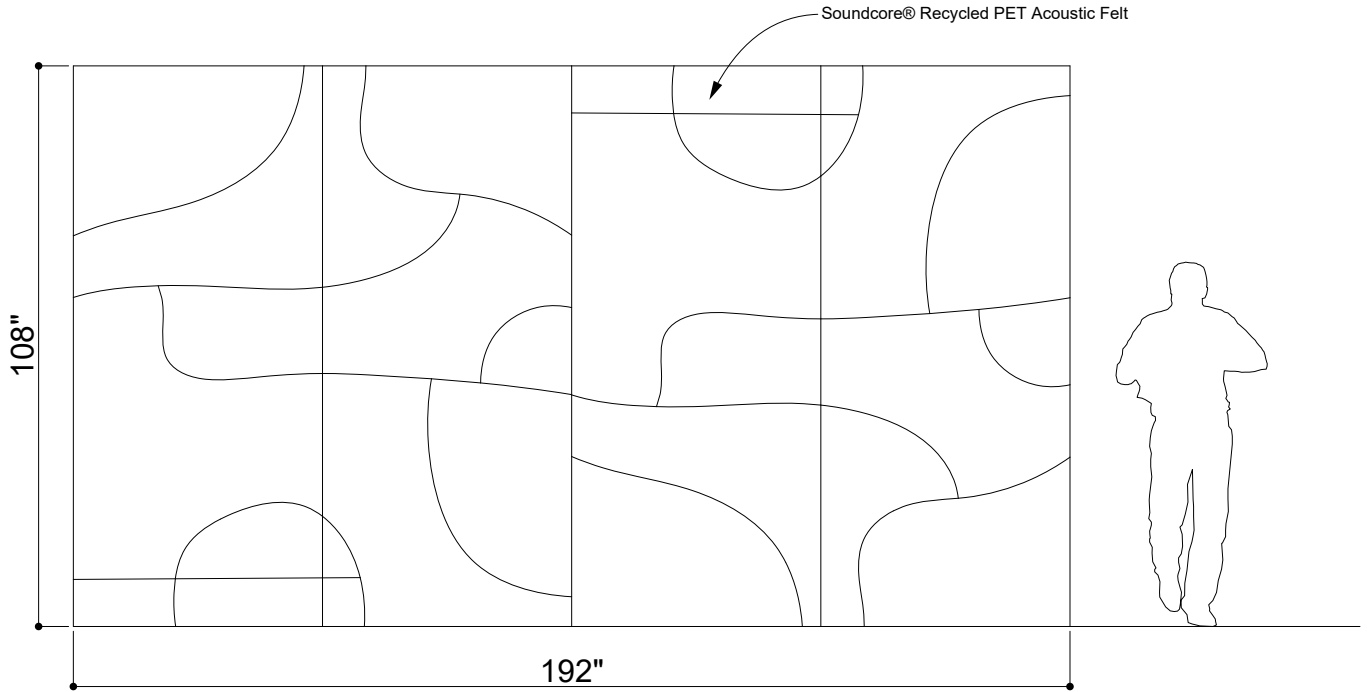
① ELEVATION 1
